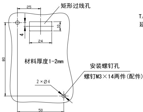
机柜安装操作面板时开孔图
