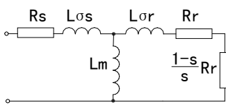
T型等效电路
