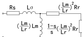
T-I型等效电路
