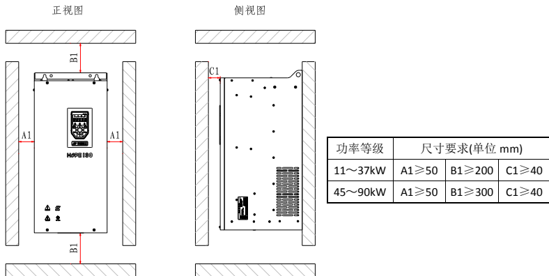
图3-2 单台机器 (Hope130G11T4~Hope130G90T4) 安装间隔
