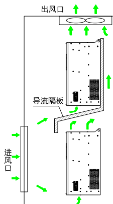
图3-4 上下排安装要求
