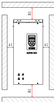
正视图
