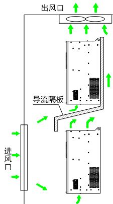
上下排安装要求
