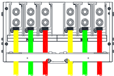
主回路输入输出端子接线效果图
