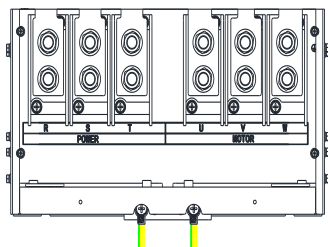
主回路接地端子接线效果图
