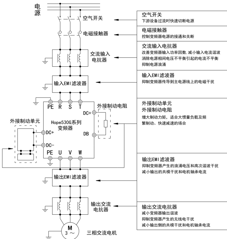
图3-8 Hope530G系列变频系统连接示意图
