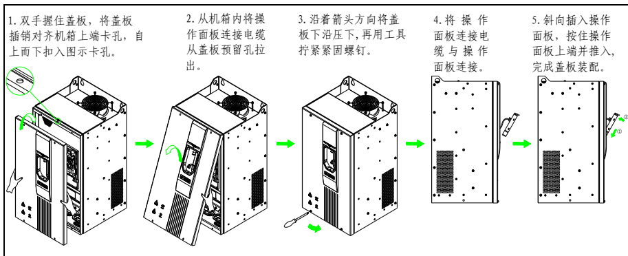
图 3-7 Hope530G18.5T6~Hope530G375T6 机型盖板拆卸与安装步骤
