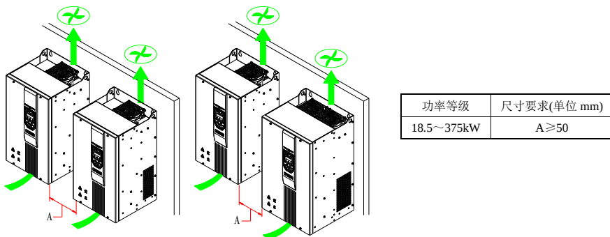
图 3-3 Hope530G18.5T6~Hope530G375T6 多台机器并排安装
