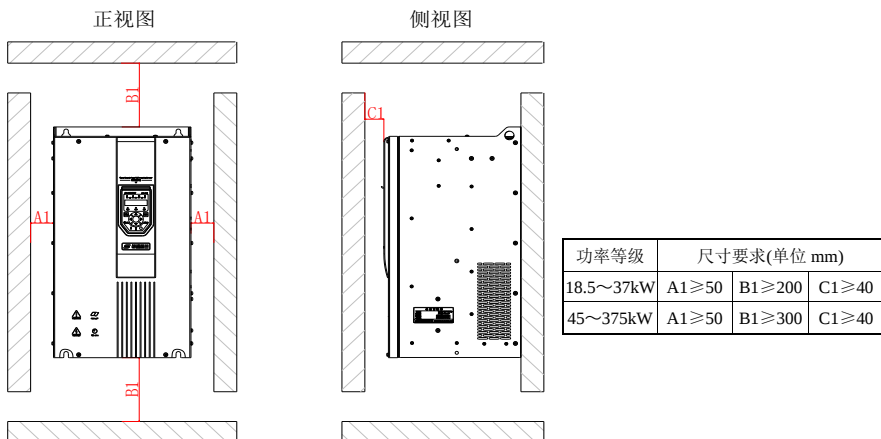
图 3-2 单台机器(Hope530G18.5T6~Hope530G375T6)安装间隔
