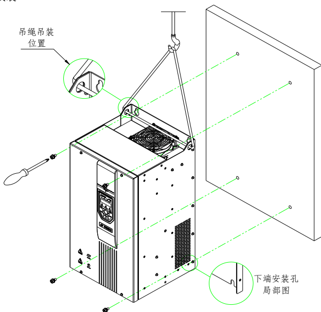
图 3-6 Hope530G18.5T6~Hope530G375T6 机型壁挂式安装
