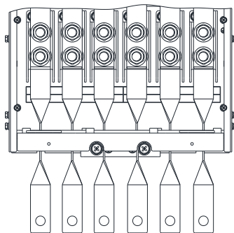
扭曲铜排在整机上接线效果示意图
