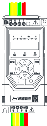
主回路接地及输入输出端子接线效果图
