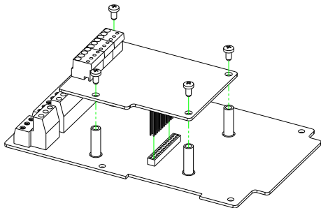
SL530-PG0在7.5kW及以下机型安装接线示意如下（SL530-PG0无需额外与控制板接线）：
