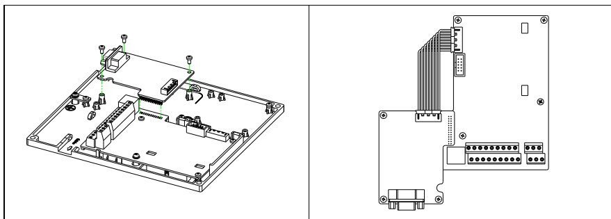
SL530-PG0在7.5kW及以下机型安装接线示意如下（SL530-PG0无需额外与控制板接线）：
