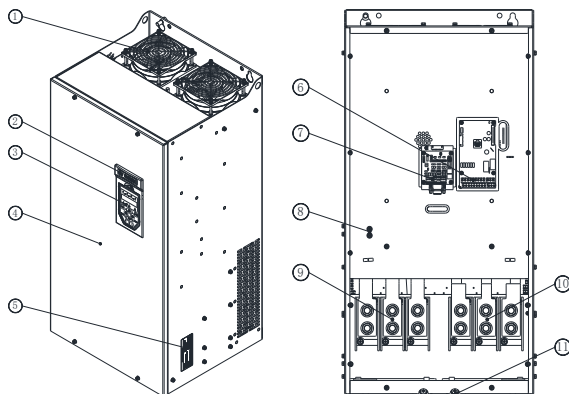
Hope130G132T4D~160T4D -产品部件示意图
