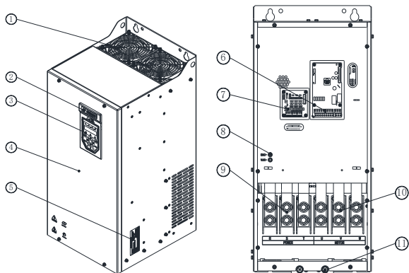
Hope130G75T4D~110T4D -产品部件示意图
