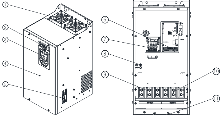
Hope130G45T4D~55T4D-产品部件示意图
