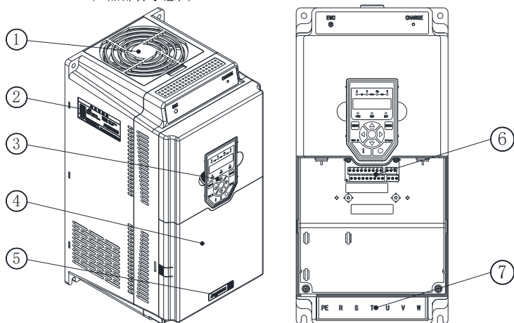
Hope130G30T4D~37T4D-产品部件示意图
