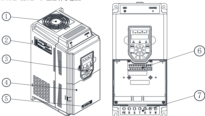
Hope130G18. 5T4D~22T4D -产品部件示意图
