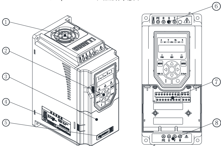
Hope130G5.5T4U~7.5T4U、Hope130G4S2U -产品部件示意图
