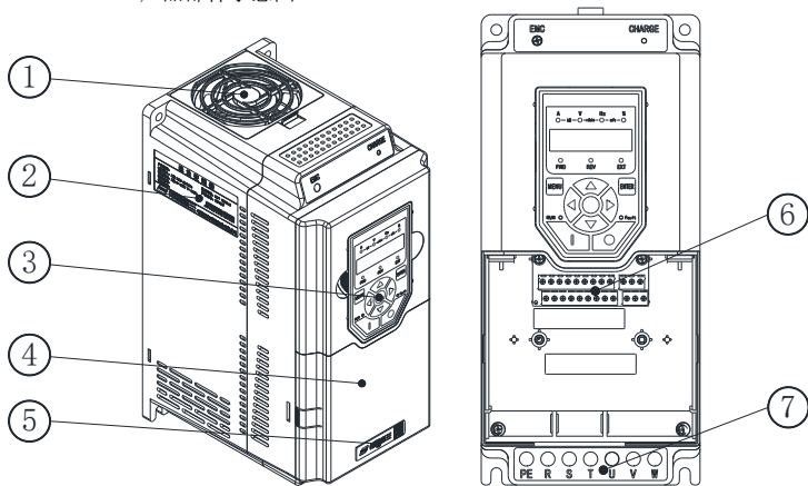
Hope130G11T4D~15T4D-产品部件示意图
