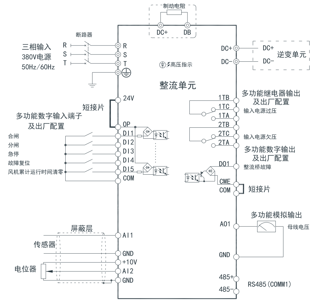
整流单元基本运行配线连接如下图
