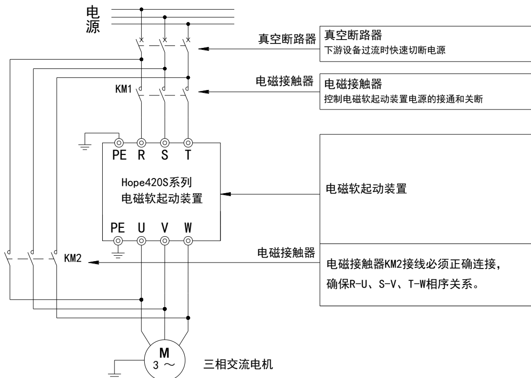
图3-9 Hope420S系列电磁软起系统连接示意图
