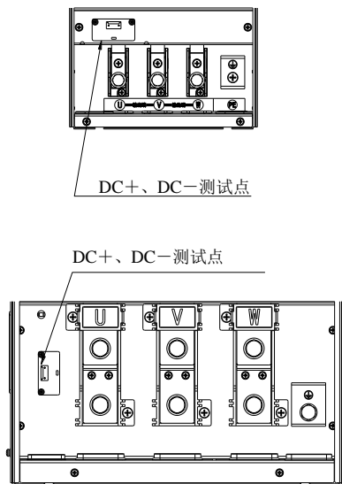
DC+、DC-参考位置图
