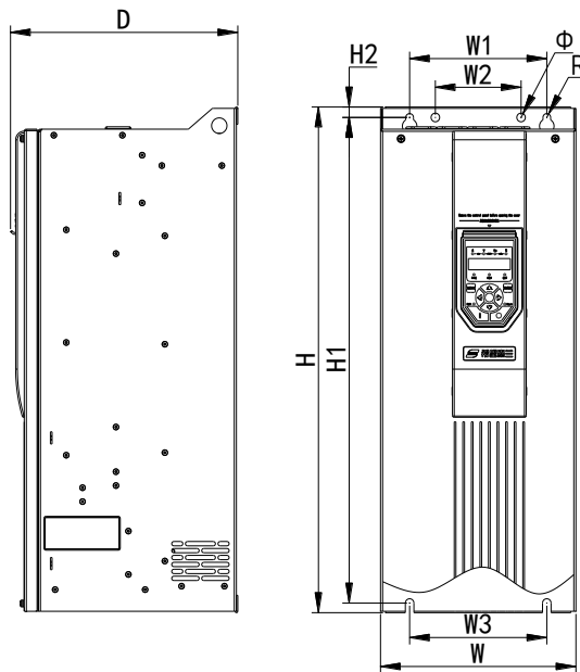
45kW~500kW 外形图
