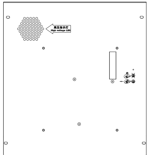
透光孔相对位置示意图
