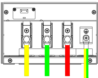
主回路端子输出端接线效果图
