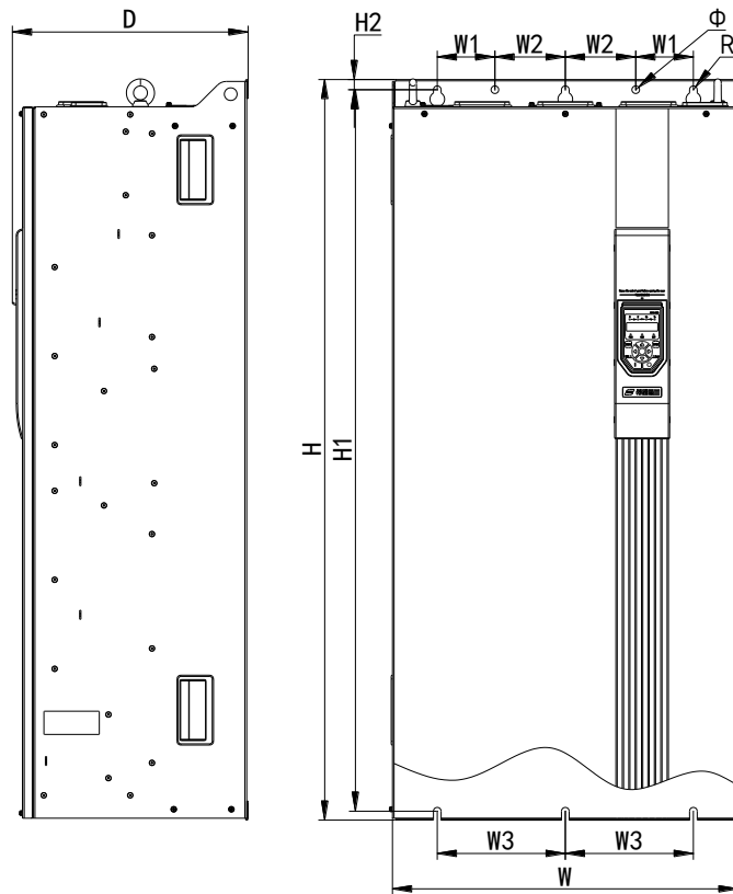
560kW~900kW 外形图
