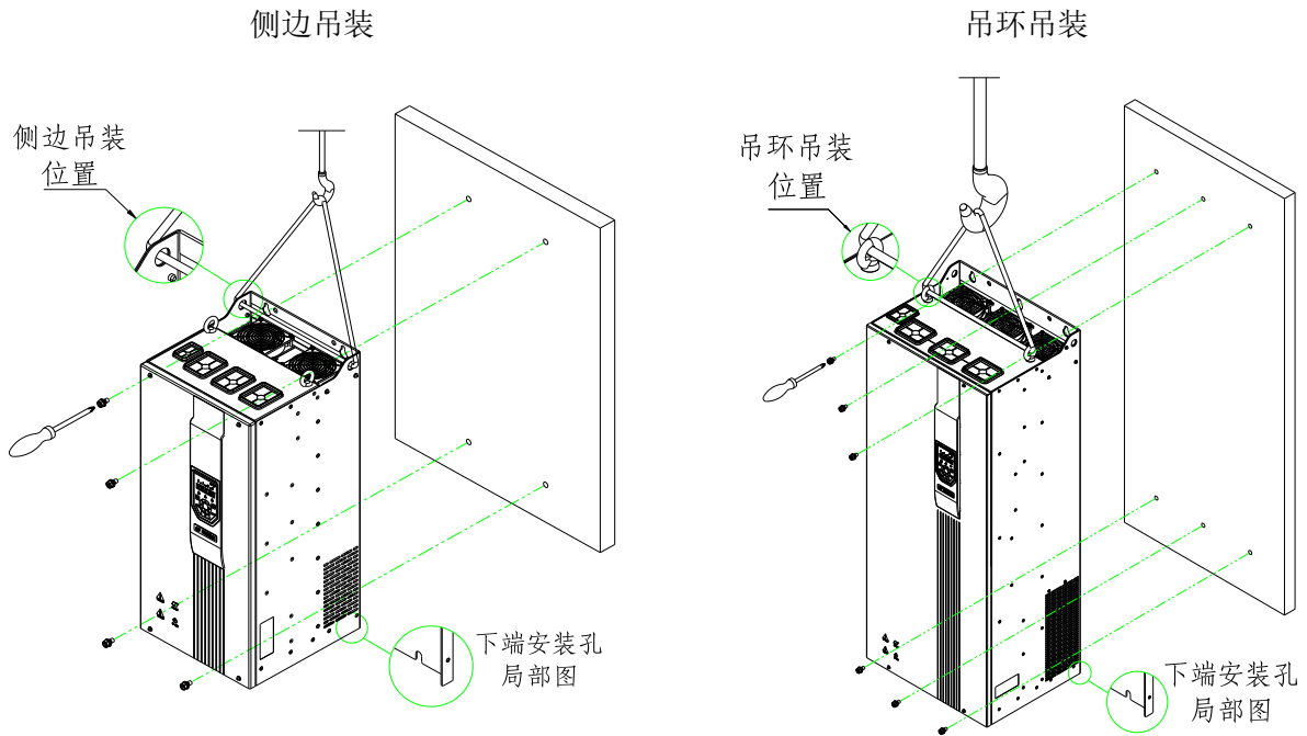
图 3-6 壁挂式安装
