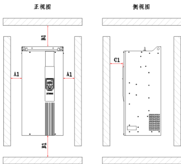
图 3-2 单台机器安装间隔
