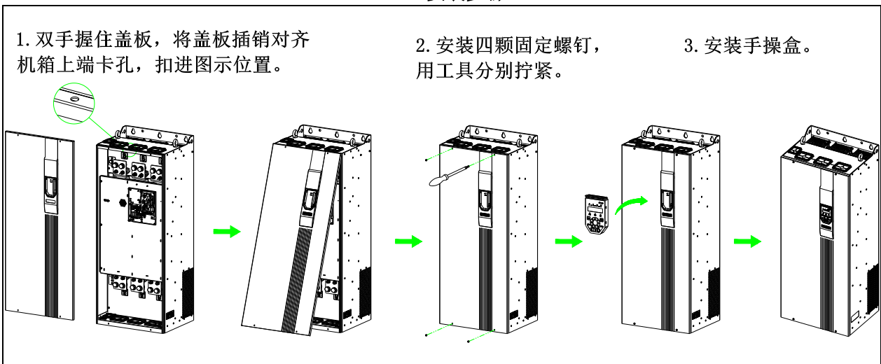
图 3-8 各机型盖板拆卸与安装步骤
