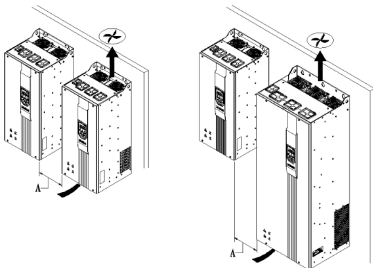
图 3-3 多台机器并排安装
