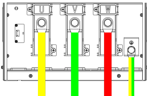
主回路端子输出端接线效果图
