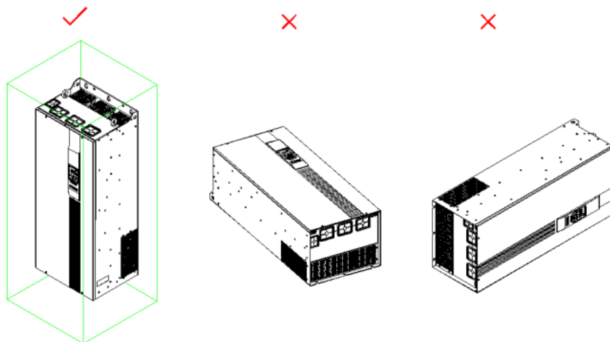
图 3-5 安装方向示意图
