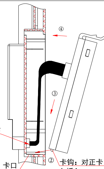
图 3-7 各机型手操盒的拆卸与安装步骤
