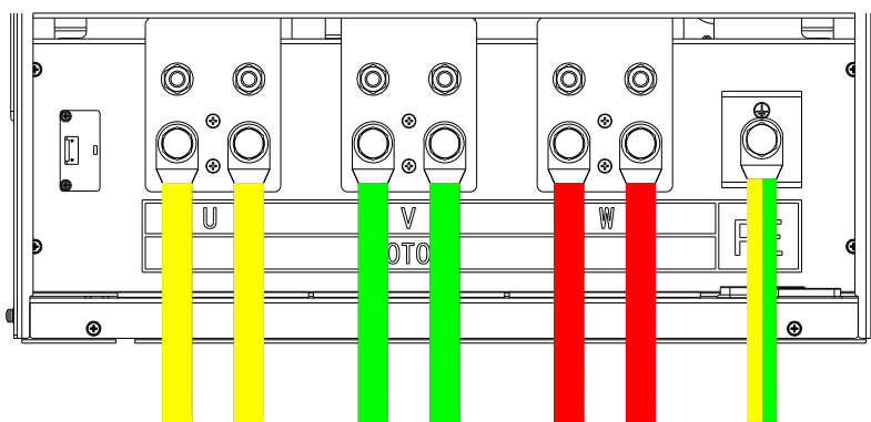
主回路端子输出端接线效果图
