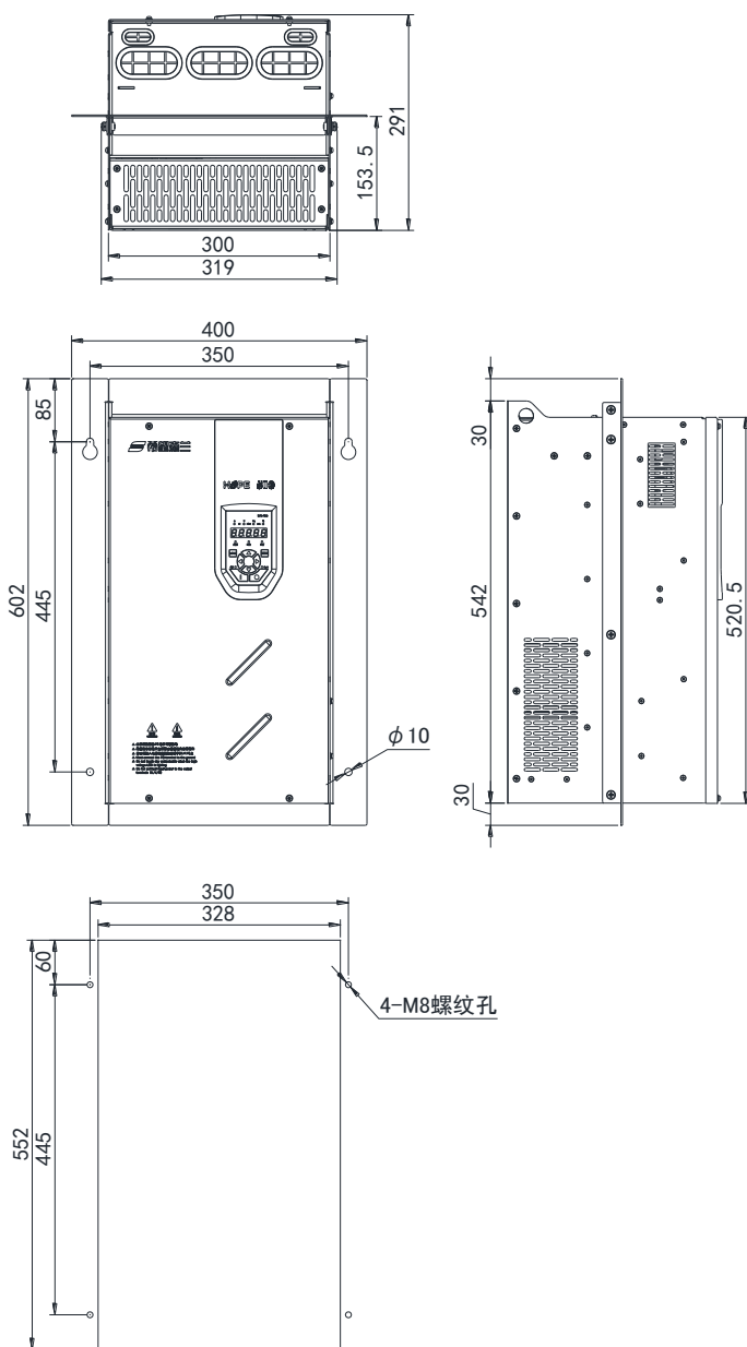
H510-A-4 安装挂条及开孔尺寸示意图
