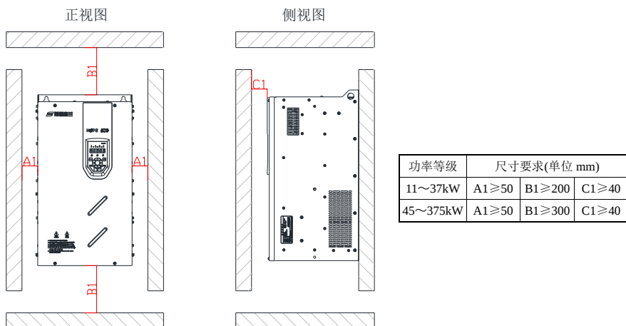
图 3-2 单台机器(Hope510G11T4~Hope510G375T4)安装间隔
