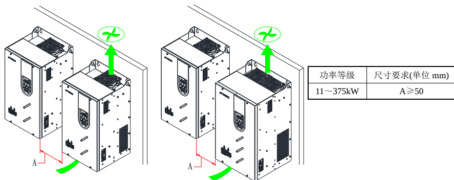
图 3-3 Hope510G11T4~Hope510G375T4 多台机器并排安装
