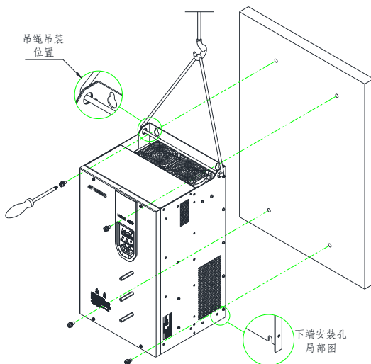
图 3-7 Hope510G45T4~Hope510G375T4 机型壁挂式安装
