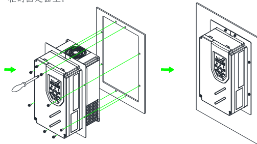
图 3-8 Hope510G11T4~Hope510G37T4 机型嵌入式安装
