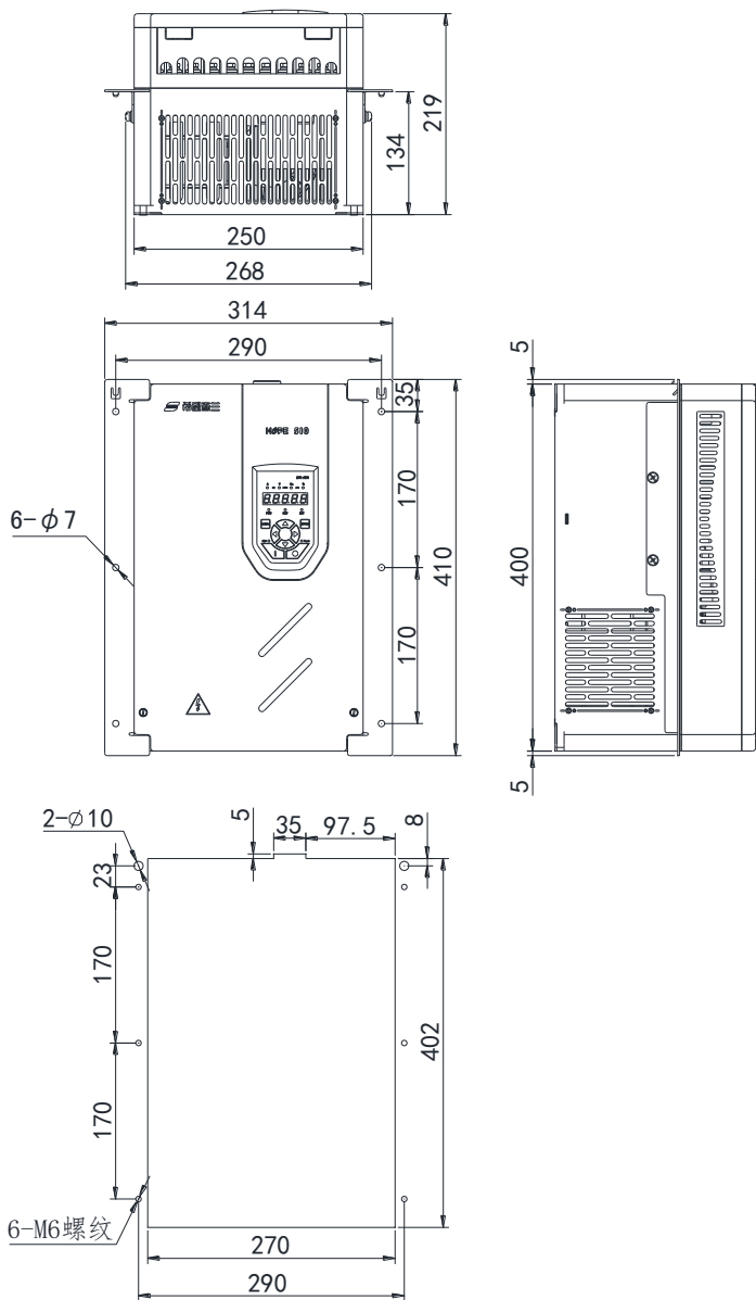
H510-A-3 安装挂条及开孔尺寸示意图
