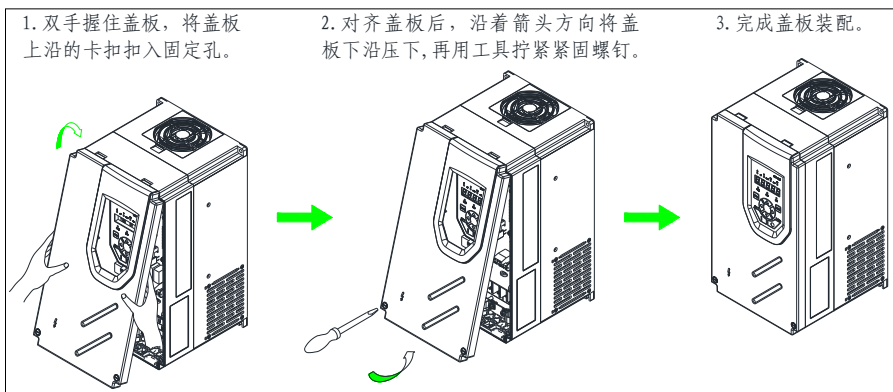
图 3-10 Hope510G11T4~Hope510G37T4 机型盖板拆卸与安装步骤
