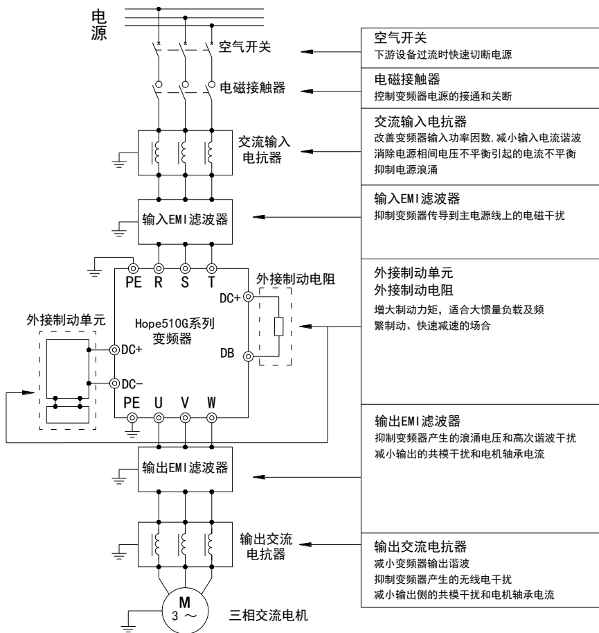
图3-12 Hope510G系列变频系统连接示意图
