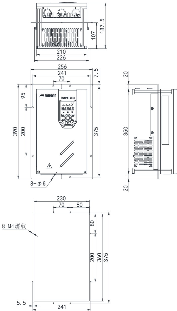
H510-A-2 安装挂条及开孔尺寸示意图
