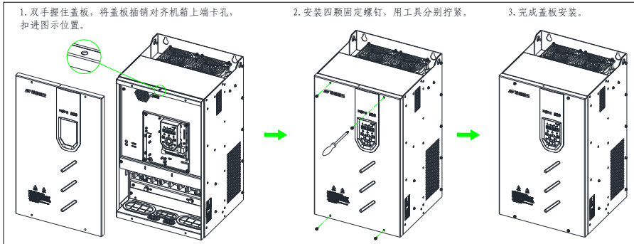
图 3-11 Hope510G45T4~Hope510G375T4 机型盖板拆卸与安装步骤
