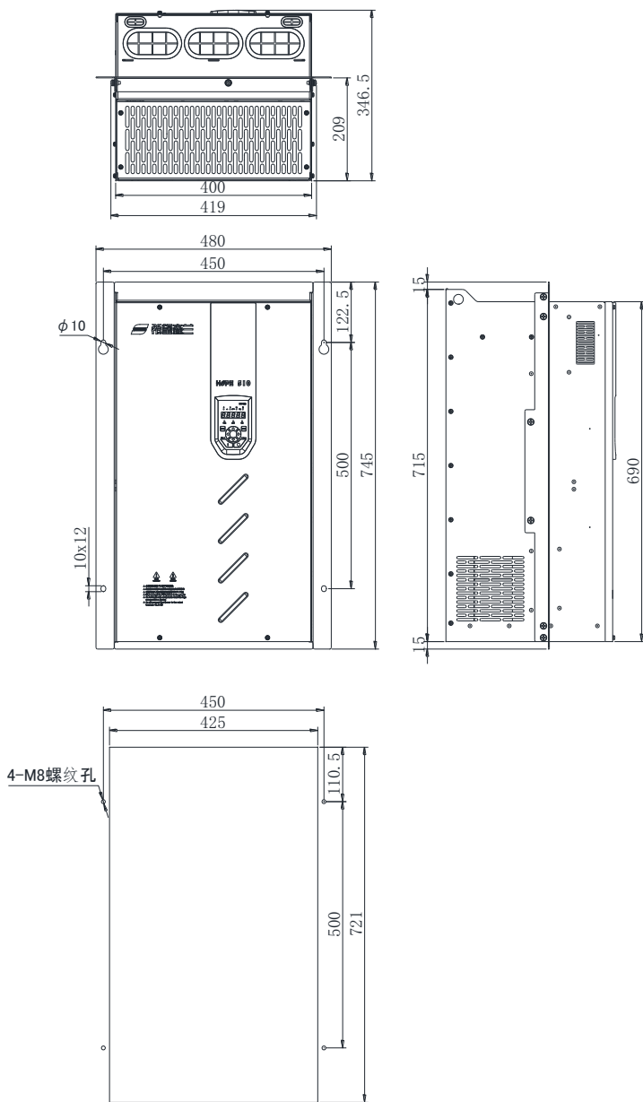
H510-A-6 安装挂条及开孔尺寸示意图
