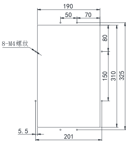
H510-A-1 安装挂条及开孔尺寸示意图
