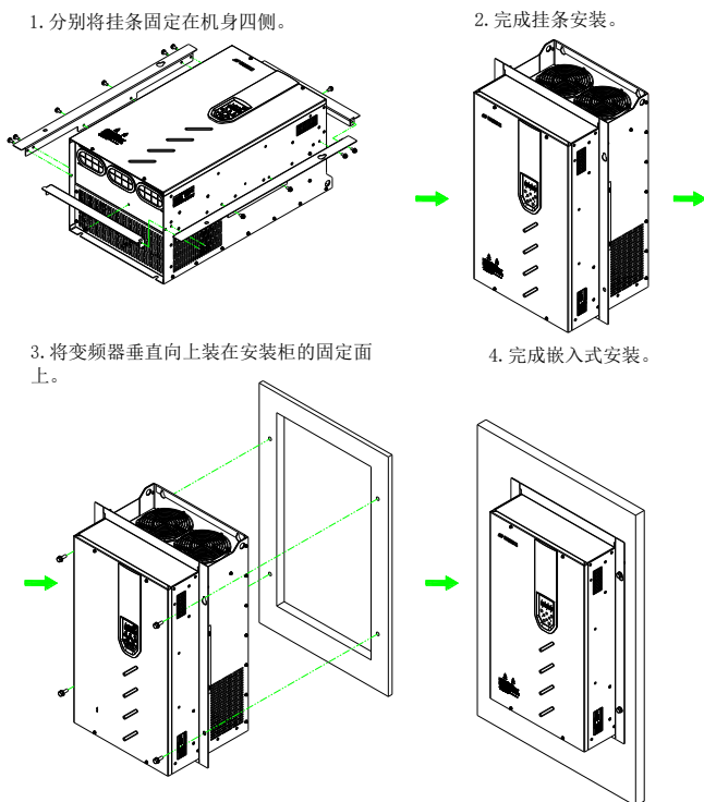
图 3-9 Hope510G45T4~Hope510G375T4 机型嵌入式安装
