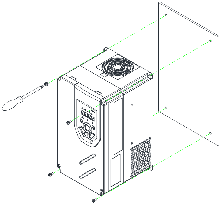
图 3-6 Hope510G11T4~Hope510G375T4 机型壁挂式安装
