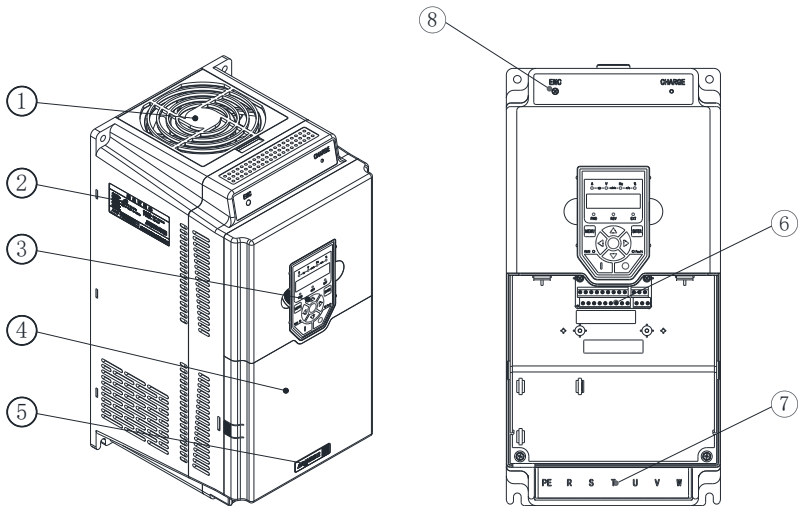
Hope150G30T4D~37T4D-产品部件示意图
