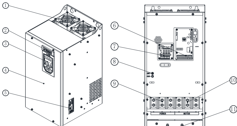
Hope150G45T4D~55T4D-产品部件示意图
