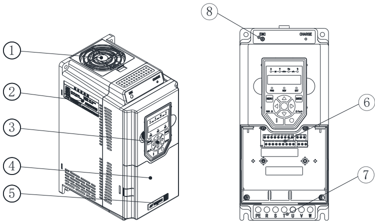
Hope150G11T4D~15T4D-产品部件示意图
