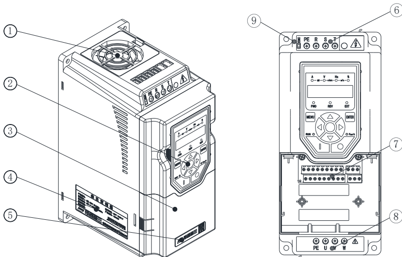
Hope150G5.5T4U~7.5T4U、Hope150G4S2U -产品部件示意图
