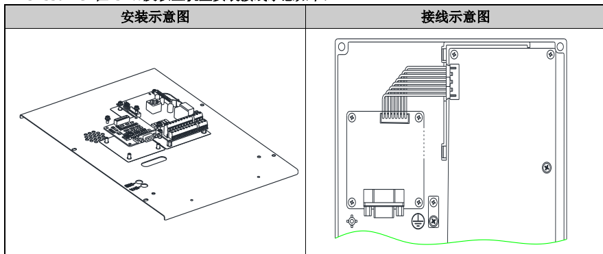
SL530-PG1在45kW及以上机型安装接线示意图如下：
