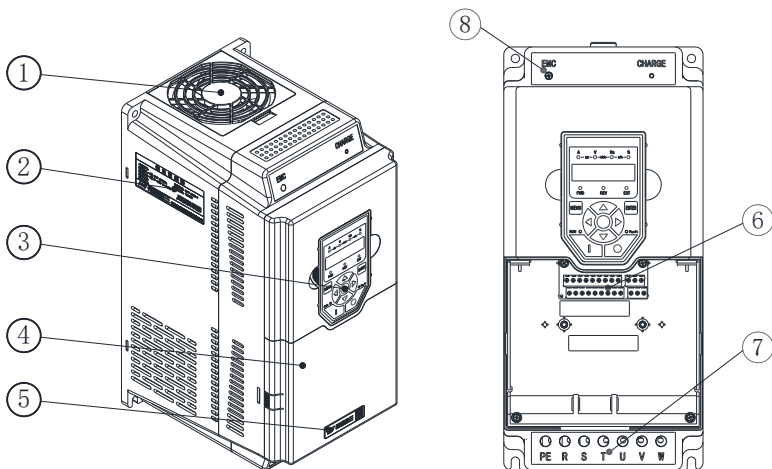
Hope150G18. 5T4D~22T4D -产品部件示意图
