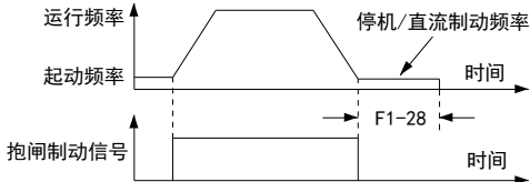
抱闸延迟时序图
