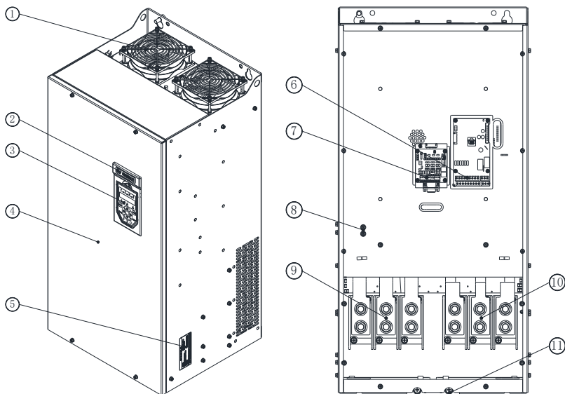
Hope150G132T4D~160T4D -产品部件示意图
