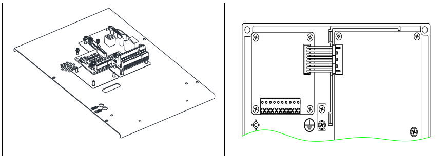
SL530-PG1在45kW及以上机型安装接线示意图如下：
