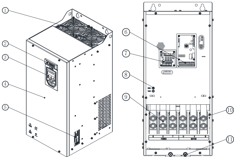
Hope150G75T4D~110T4D -产品部件示意图
