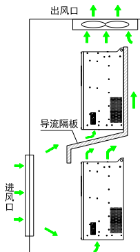
上下排安装要求
