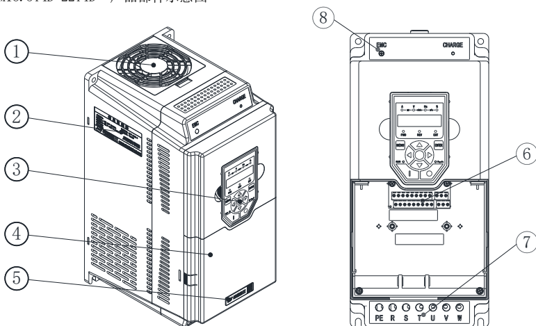
Hope150PM18. 5T4D~22T4D -产品部件示意图
