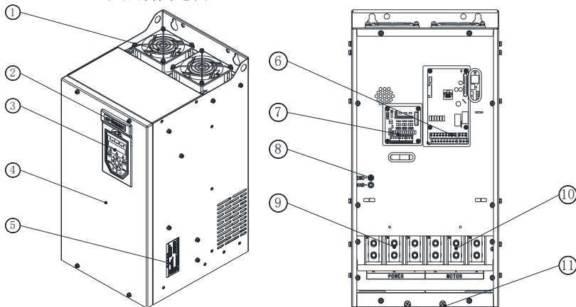
Hope150PM45T4D~55T4D-产品部件示意图
