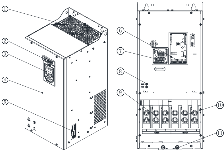
Hope150PM75T4D~110T4D 产品部件示意图
