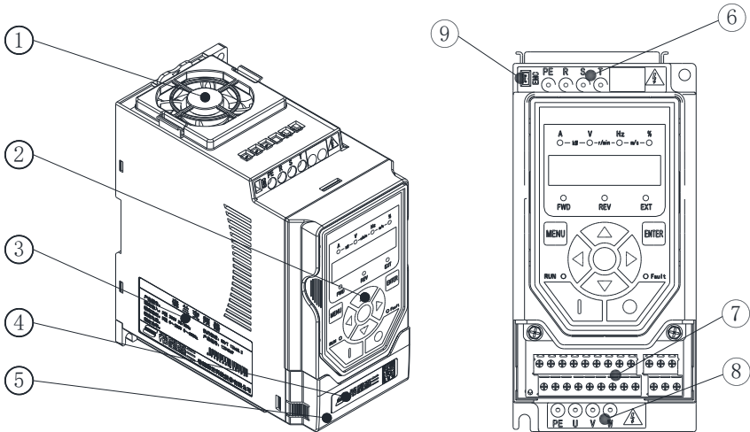
Hope150PM0.75T4U~4T4U、0.55S2U~2.2S2U -产品部件示意图
