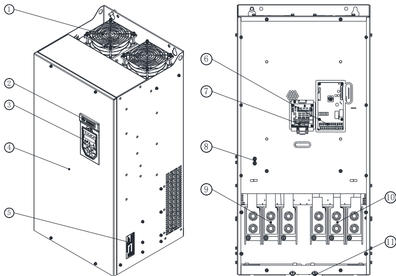
Hope150PM132T4D~160T4D -产品部件示意图
