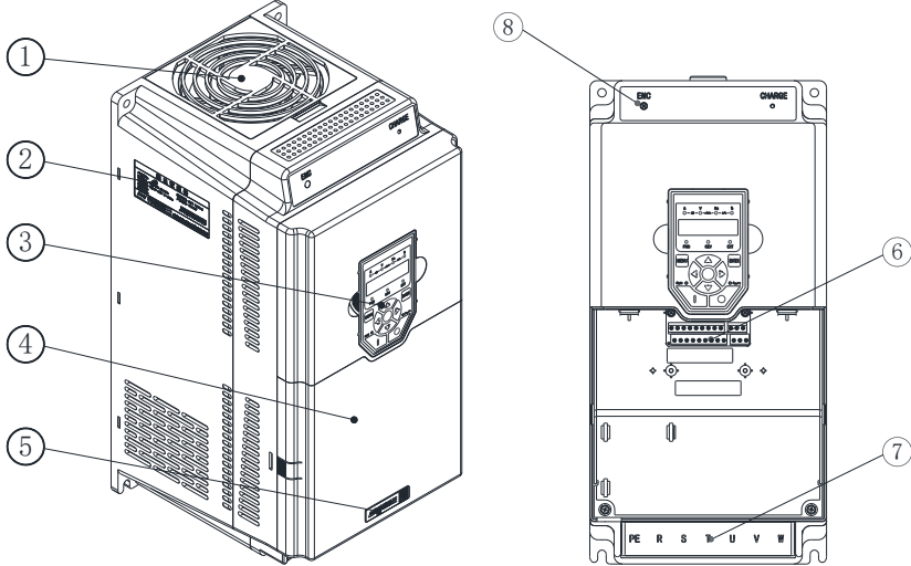
Hope150PM30T4D~37T4D-产品部件示意图
